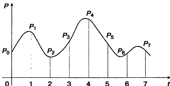
Рис. 1.9. Барограмма
